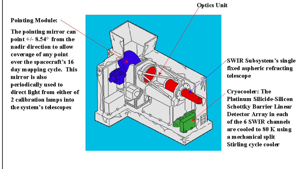
Εικόνα του καταγραφικού συστήματος SWIR
